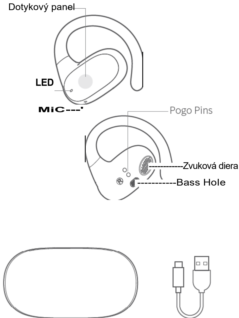
Nabíjacia schránka
